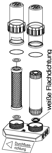
Bild 1: Einbau im DUO-HP
