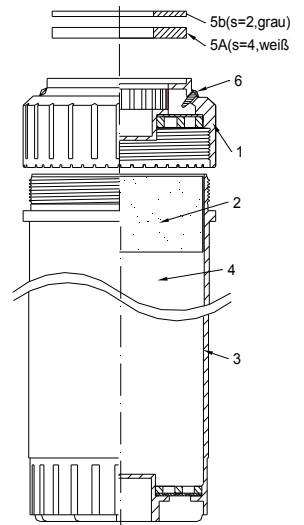
Bild 4: Ionentauscherkartusche
