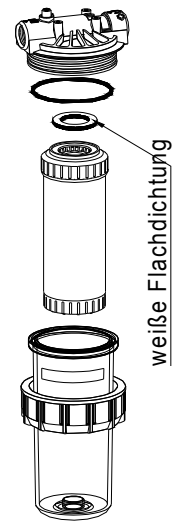
Bild 2 : Einbau im Vario-HP
